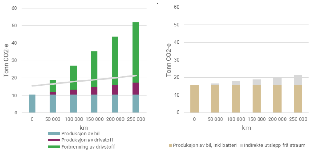
Figur 2: Samanlikning av klimafotavtrykket til ein tung elbil og ein tilsvarande bil med forbrenningsmotor. Elbilen har eit større avtrykk frå produksjon, men mindre utslepp knytt til drift.
